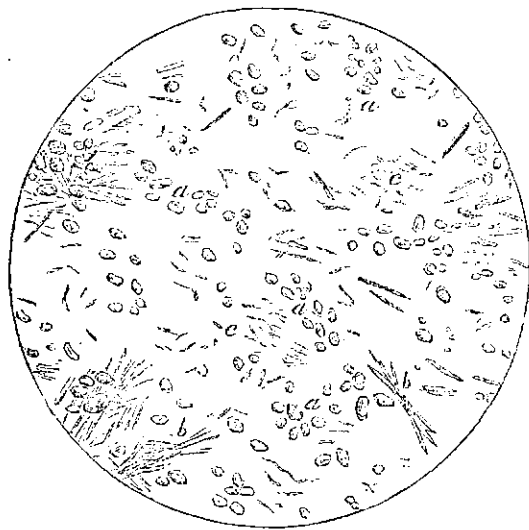
a. Fermento alcohólico del vino. b. Cristales de bitartrato de potasa.
