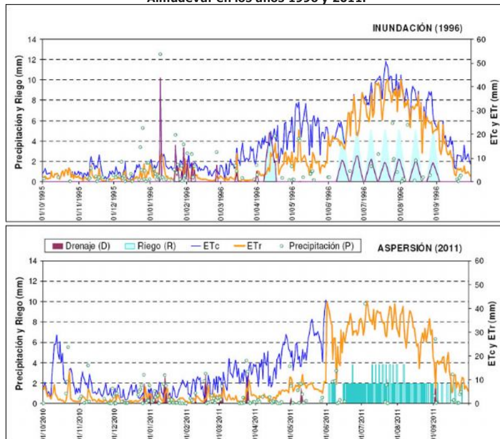
Figura 2. Evolución diaria de los principales términos del balance de agua en el suelo para el cultivo de maíz en Almodóvar en los años 1996 y 2011.
