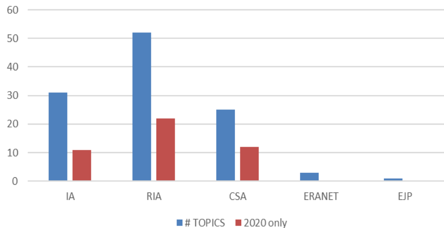
# TOPICS 2018-2020
