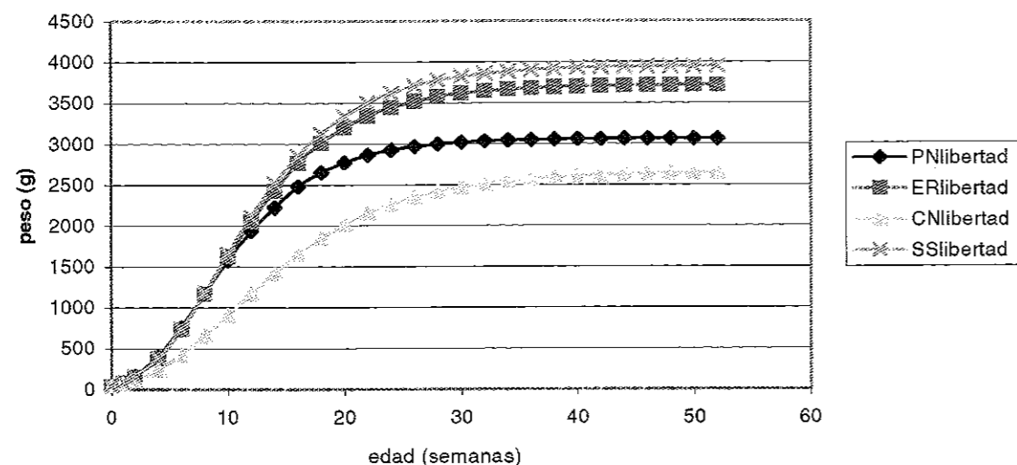
Figura 2. Curvas de crecimiento, estimadas según el modelo, para los pollos criados en libertad. Figure 2. Growth curves, estimate according to the model, for the chickens bred in free-range.
