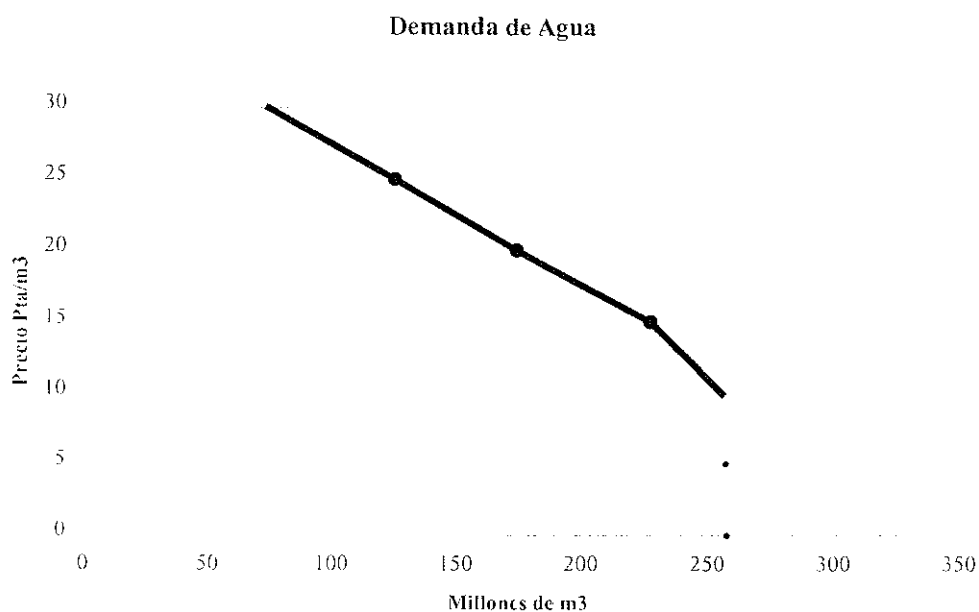
Figura 2 Demanda de agua en el sistema Flumen-Monegros
