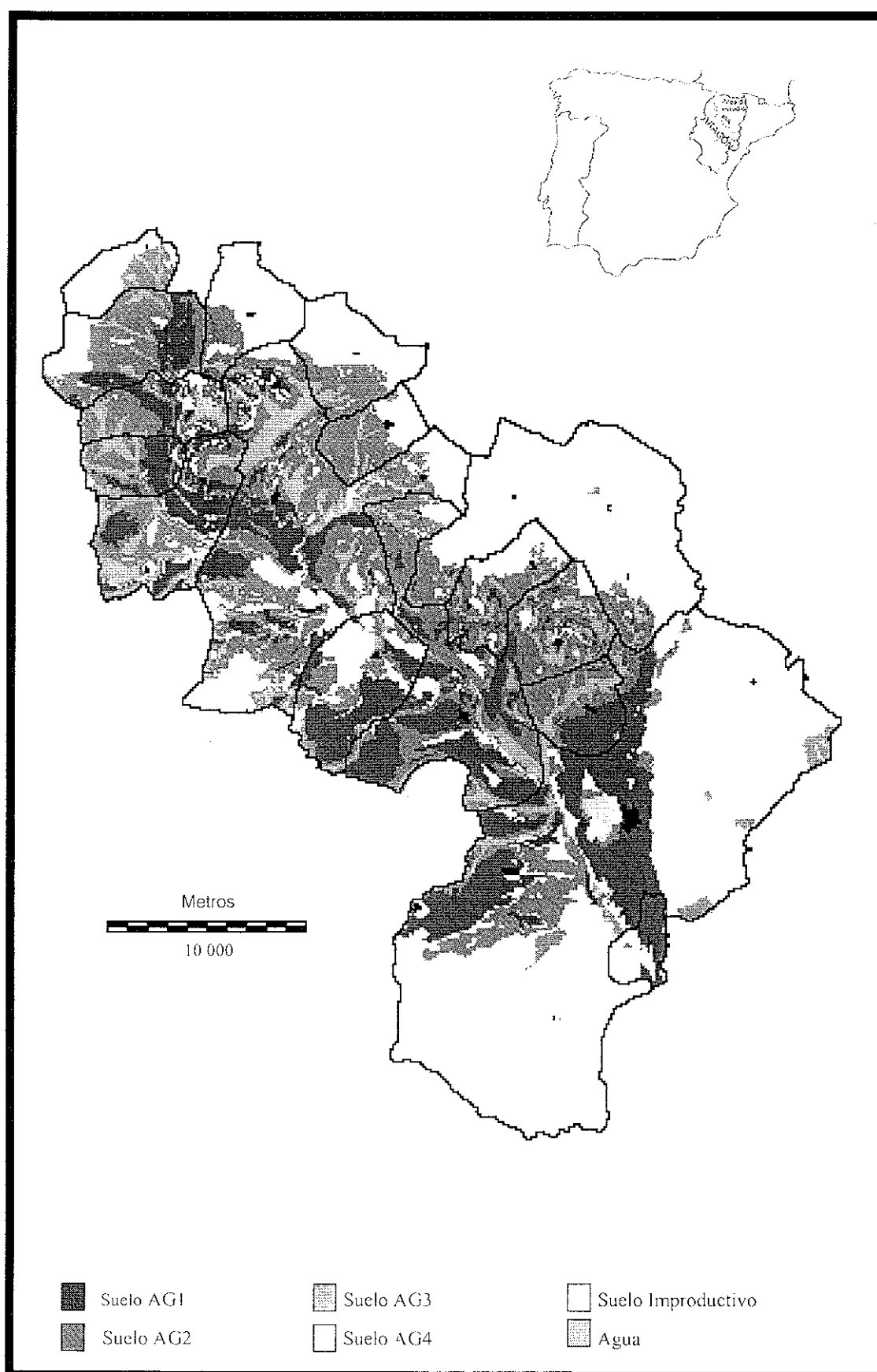
Figura 1 Mapa de tipos de suelo en el regadío Flumen-Monegros
