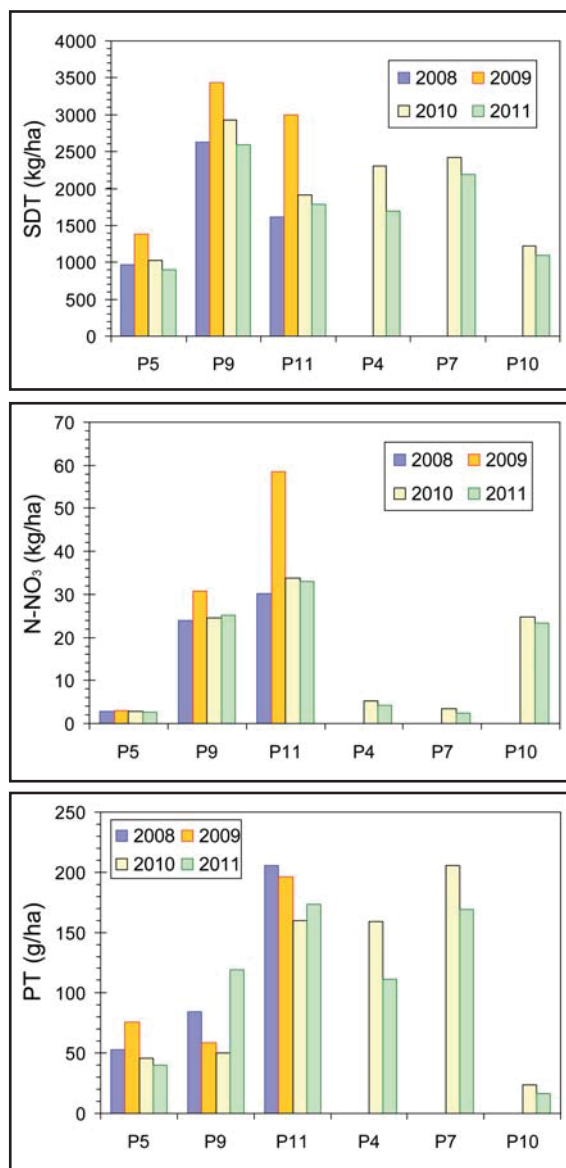
Figura 2. Masas exportadas de sales (SDT), nitrógeno nítrico (N-NO 3 ) y fósforo total (PT) por unidad de superficie regada en las cuencas de estudio en los años hidrológicos 2008 a 2011.
